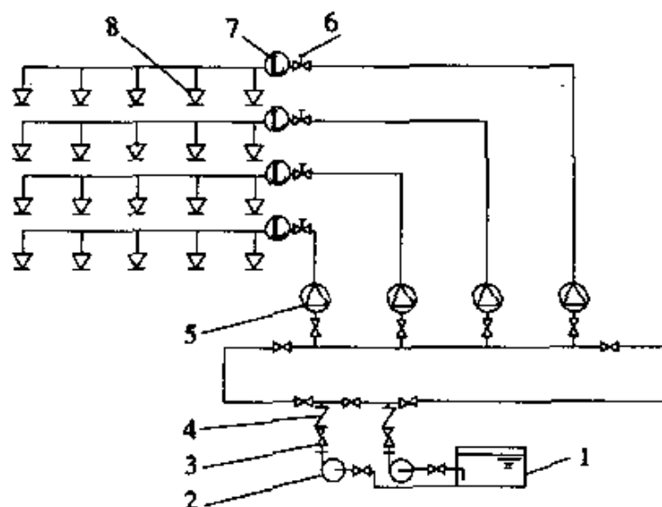
图 24 环状供水示意图
